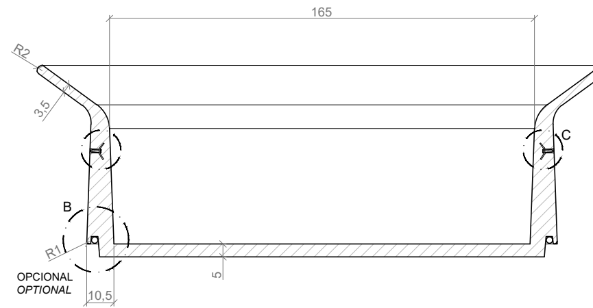
SECCION A-A' / SECTION A-A'
