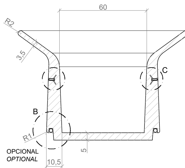
SECCION A-A' / SECTION A-A'
