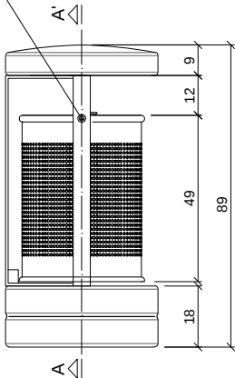
PERFIL / PROFIL VIEW
