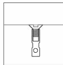
Detalle casquillo Tapón de acero inox
