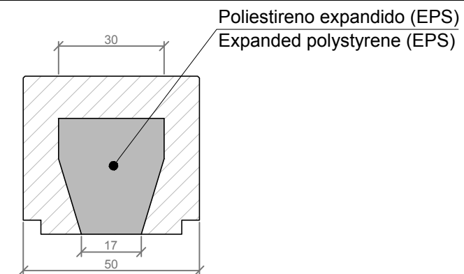
SECCION B-B' / SECTION B-B'
