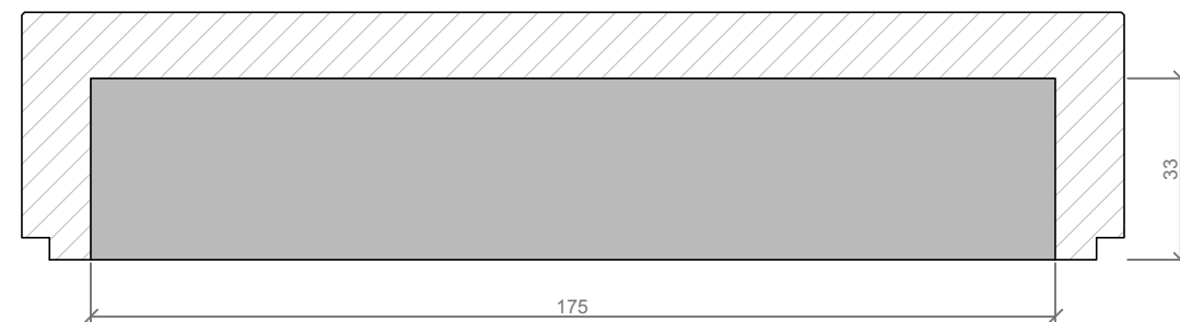
SECCION A-A' / SECTION A-A'
