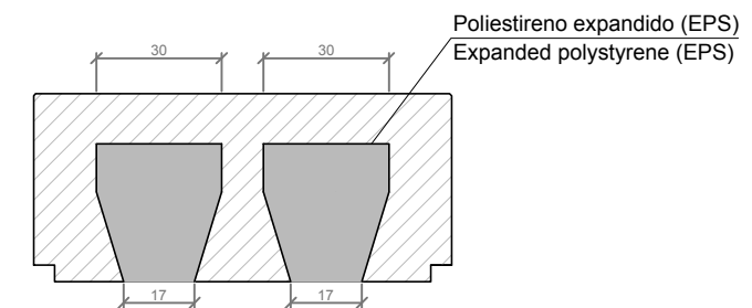
SECCION B-B' / SECTION B-B'
