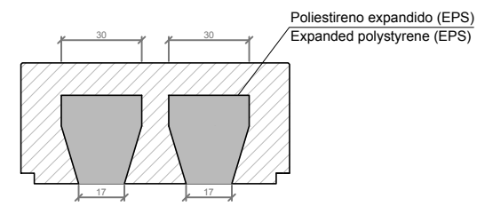
SECCION B-B' / SECTION B-B'
