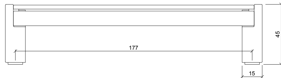
ALZADO
