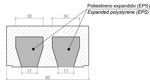
SECCION B-B' / SECTION B-B'
