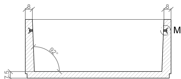
SECCION A-A' / SECTION A-A'
