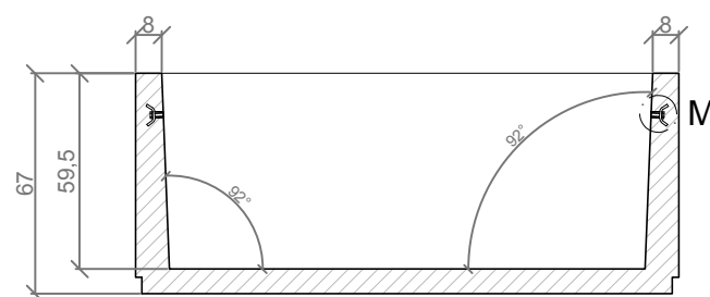
SECCION B-B' / SECTION B-B'
