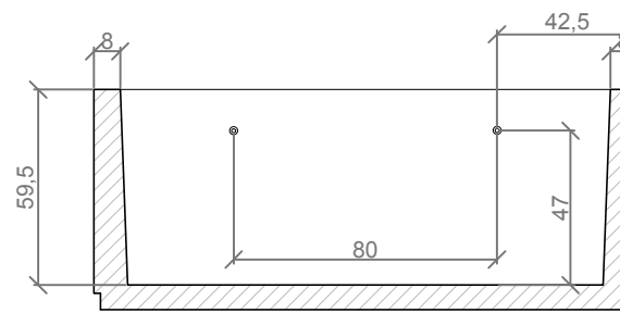
SECCION C-C' / SECTION C-C'
