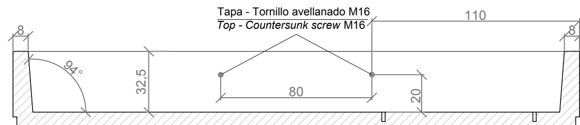
SECCION A-A' / SECTION A-A'
