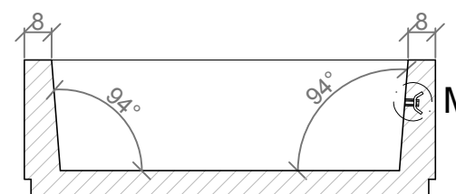
SECCION B-B' / SECTION B-B'
