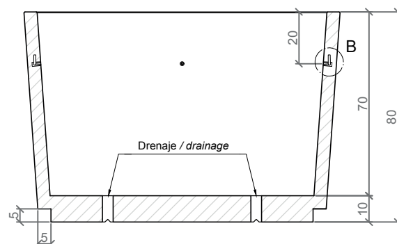
SECCION A-A' / SECTION A-A'
