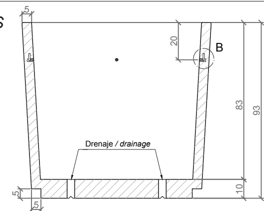
SECCION A-A' / SECTION A-A'
