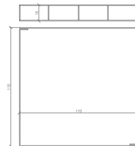
ALZADO DETALLE E ALZADO DETAIL E
