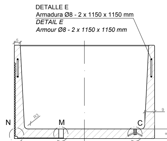
SECCION A-A' / SECTION A-A'
