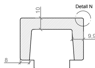
SECCION / SECTION
