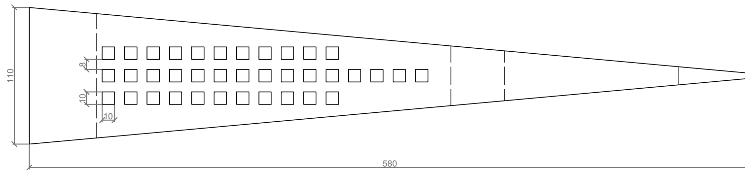
PLANTA / TOP VIEW
