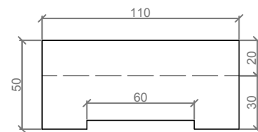
ALZADO IZQUIERDO / LEFT VIEW
