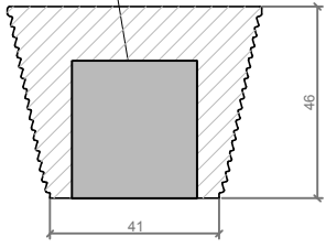
SECCION B-B' / SECTION B-B'
