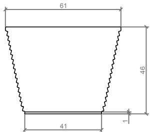
PERFIL / PROFILE
