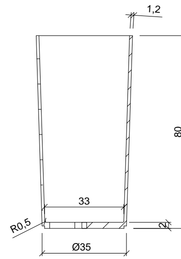
SECCION A-A
