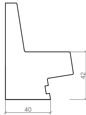
PERFIL / RIGHT VIEW
