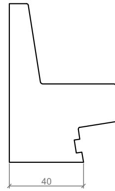
PERFIL / PROFILE
