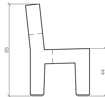
PERFIL / PROFILE
