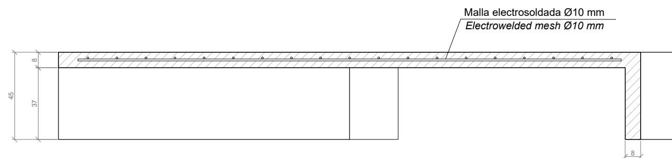
SECCION / SECTION
