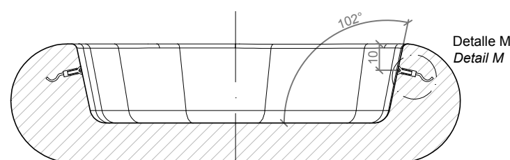
SECCION / SECTION
