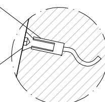
DETALLE M / DETAIL M Casquillo de elevación / Lifting sleeve
